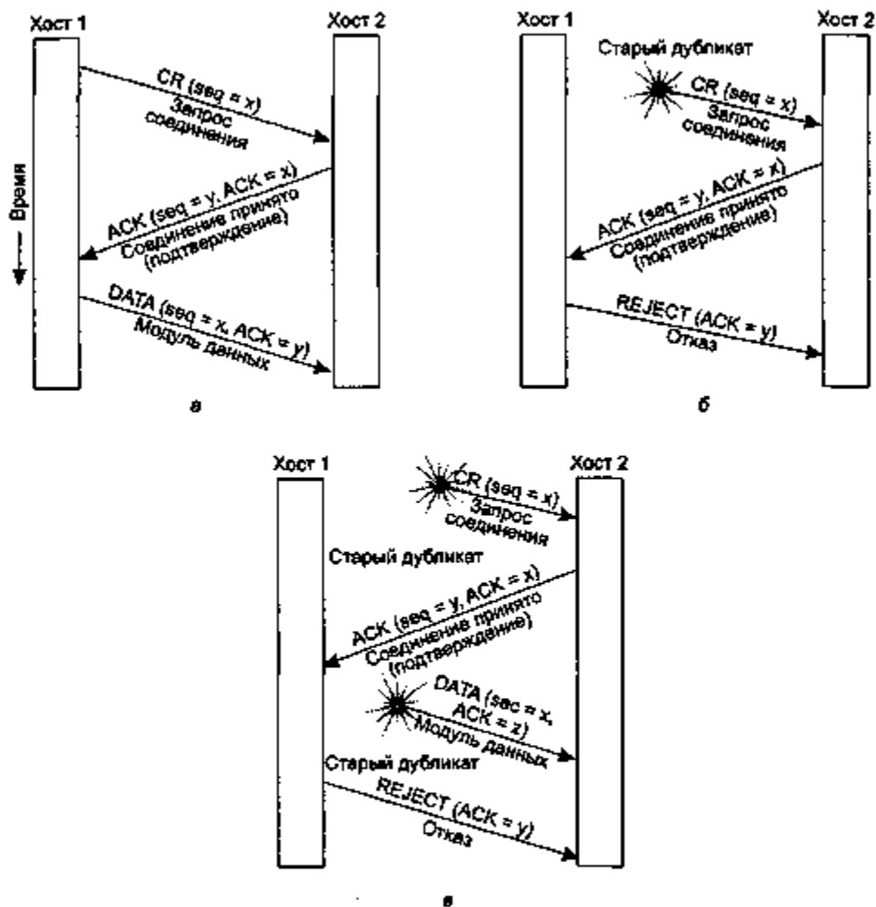
Рис. 6.8. Три сценария установки соединения с помощью «тройного рукопожатия». CR означает CONNECTION REQUEST. Нормальная работа (а); появления старого дубликата CONNECTION REQUEST (б); дубликат модуля CONNECTION REQUEST и дубликат модуля ACK (в)
