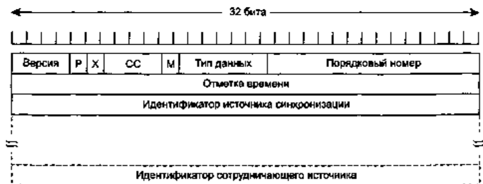
Рис. 6.21. Заголовок RTP
