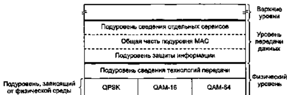
Рис. 4.26. Стек протоколов 802.16
