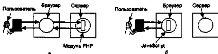
Рис. 7.16. PHP-скрипт на стороне сервера (а); сценарий на JavaScript на стороне клиента (б)
