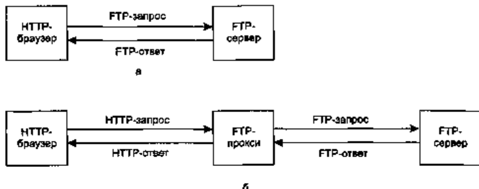
Рис. 8.25. Брандмауэр, состоящий из двух пакетных фильтров и шлюза прикладного уровня
