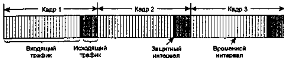
Рис. 4.30. Дуплексная связь с временным разделением: кадры и временные интервалы
