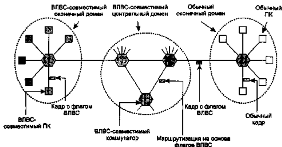
Рис. 4.46. Передача данных из обычного Ethernet в ВЛВС-совместимый Ethernet. Затененные символы — это ВЛВС-устройства. Все остальные несовместимы с виртуальными сетями
