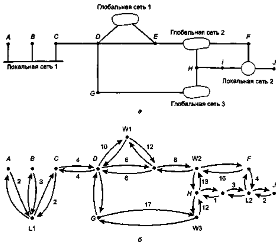
Рис. 5.35. Автономная система (а); представление а в виде графа (б)
