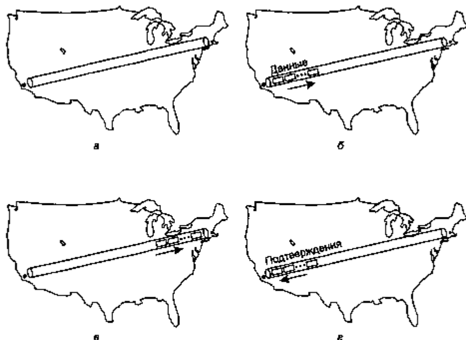
Рис. 6.34. Первая половина мегабита из Сан-Диего в Бостон: в момент времени t = 0 (а); через 500 мкс (б); через 20 мс (в); через 40 мс (г)
