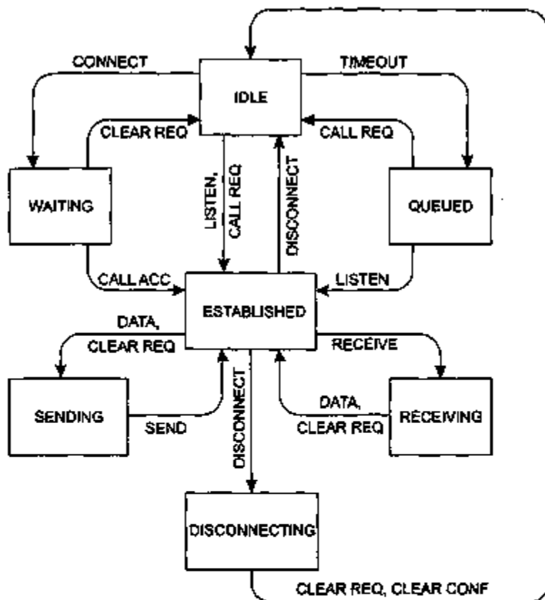
Рис. 6.17. Пример протокола в виде графа. Для простоты переходы, не изменяющие состояния соединения, были опущены
