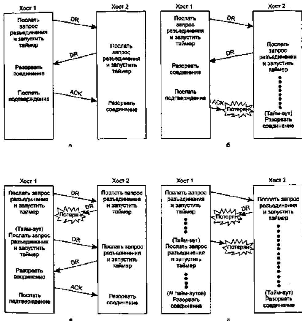
Рис. 6.11. Четыре сценария разрыва соединения: нормальный случай «тройного рукопожатия» (а); потеряю последнее подтверждение (б); потеря ответ (в); потеря ответ и последующие запросы (г)
