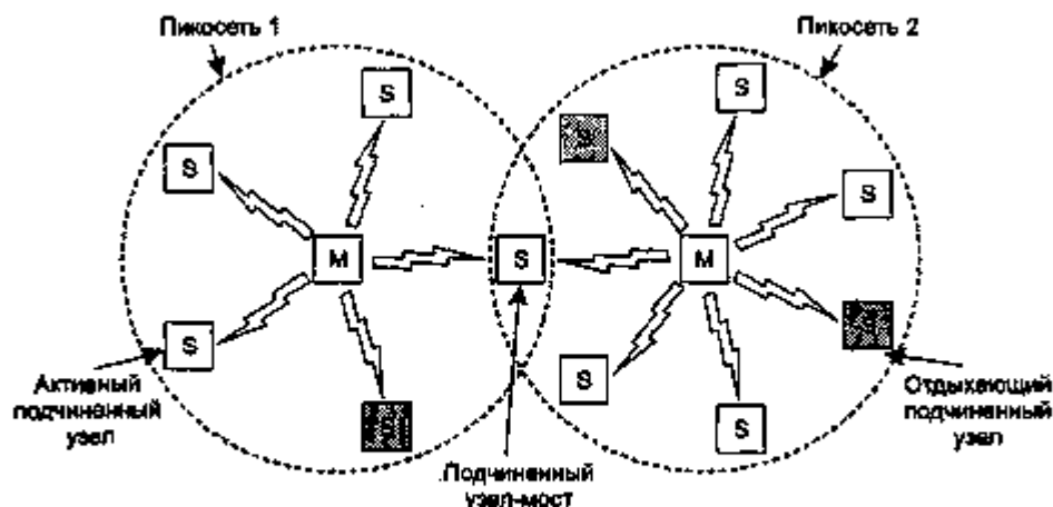
Рис. 4.32. Два пикосети могут, соединившись, сформировать рассеянную сеть
