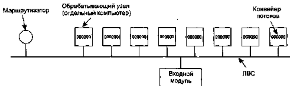
Рис. 7.10. Серверная ферма
