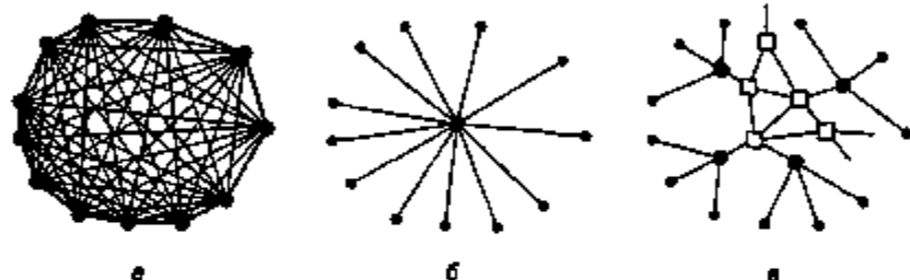
Рис. 2.16. Сеть «каждый с каждым» (а); централизованный коммутатор (б); двухуровневая иерархия (в)
