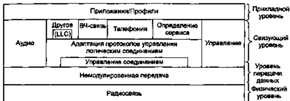
Рис. 4.93. Архитектура протоколов Bluetooth; версия 802.15
