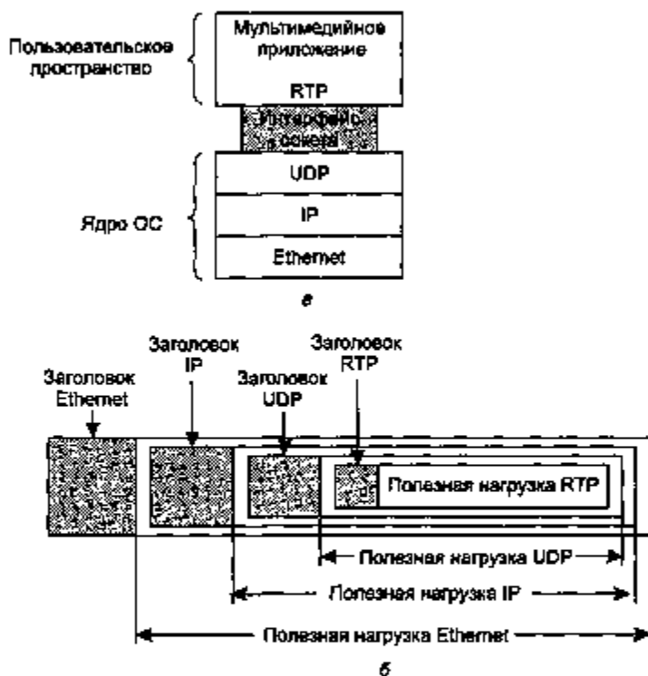
Рис. 6.20. Положение RTP в стеке протоколов (а); вложение пакетов (б)
