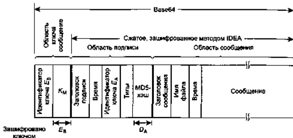
Рис. 8.41. PGP-сообщение
