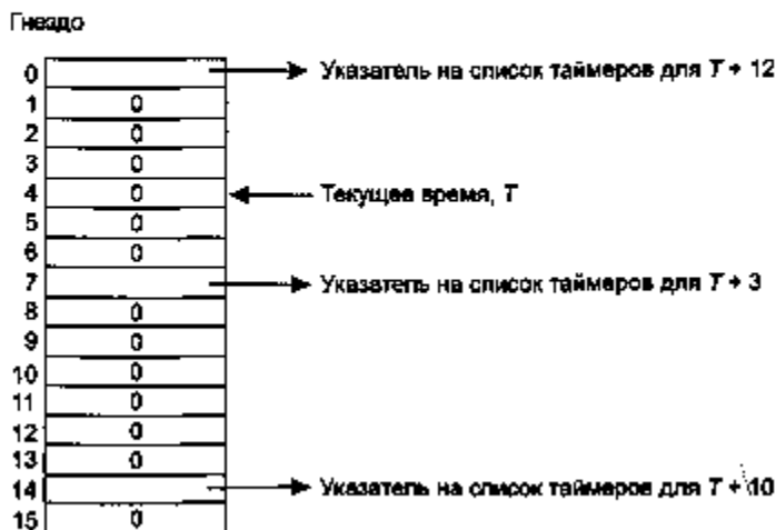
Рис. 6.39. Колесо времени
