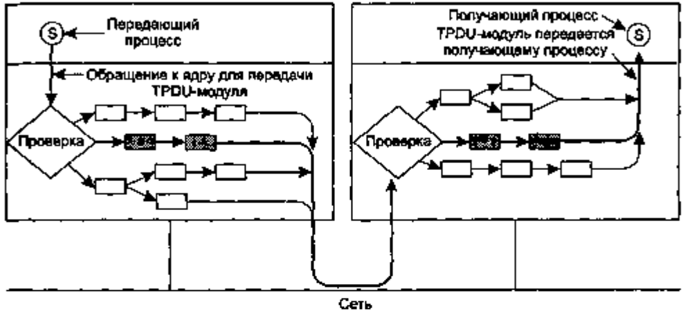
Рис. 6.37. Быстрый путь от отправителя до получателя показан жирной линией. Шаги обработки вдоль этого пути показаны заштрихованными прямоугольниками
