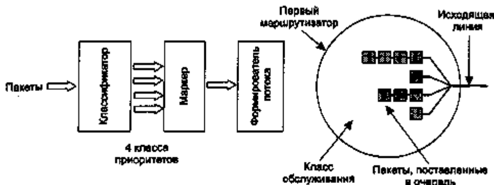
Рис. 6.35. Возможная реализация гарантированной пересылки потока данных
