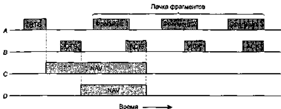
Рис. 4.25. Пачка фрагментов
