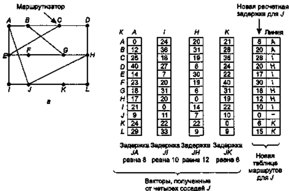
Рис. 5.7. Подсеть (а); полученные от A, I, H и K векторы и новая таблица маршрутов для J (б)
