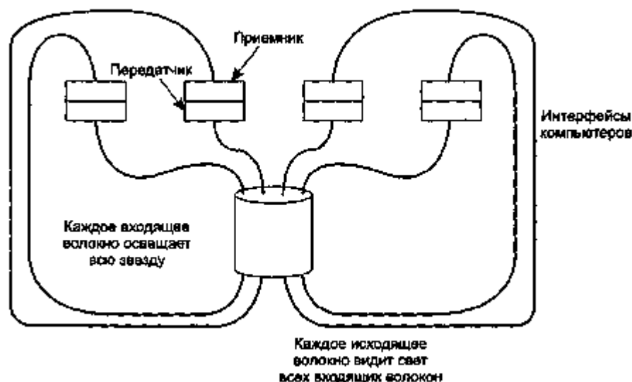
Рис. 2.8. Соединение типа «пассивная звезда» в оптоволоконных сетях
