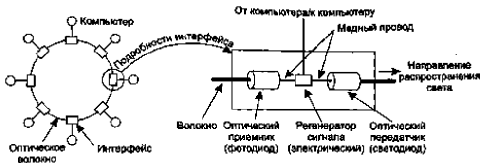
Рис. 2.7. Оптоволоконное кольцо с активными повторителями
