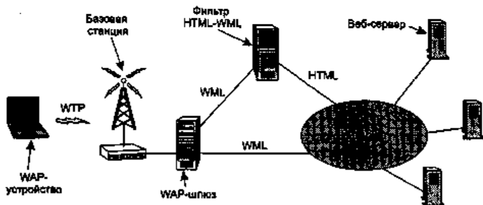
Рис. 7.21. Архитектура WAP
