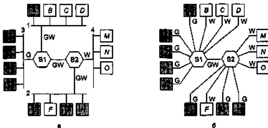
Рис. 4.45. Четыре физические ВЛС, объединенные в две виртуальные сети, серую и белую, двумя мостами (а); те же 15 машин, объединенных в две виртуальные сети коммутаторами (б)
