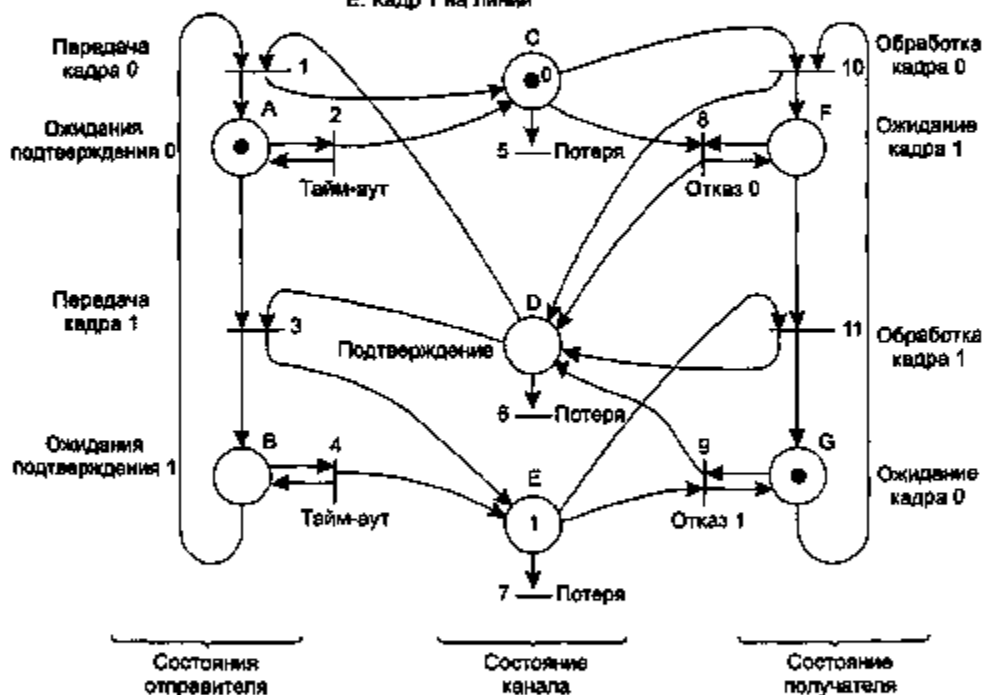
Рис. 3.16. Сетевая модель Петри для протокола 3
