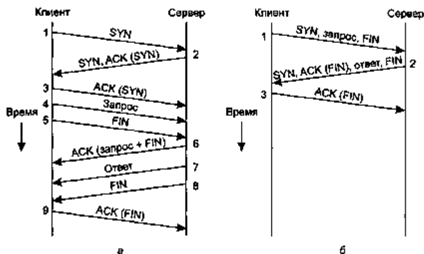
Рис. 6.33. Удаленный вызов процедуры с помощью обычного TCP (а); удаленный вызов процедуры с помощью T/TCP (б)
