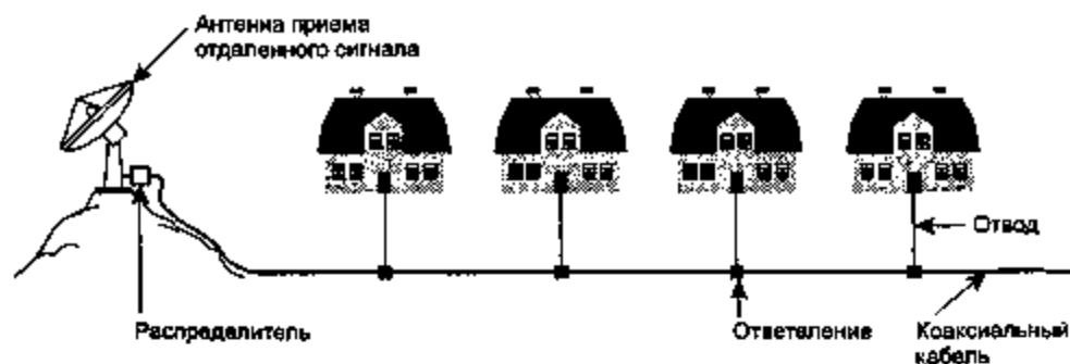
Рис. 2.40. Первая система кабельного телевидения
