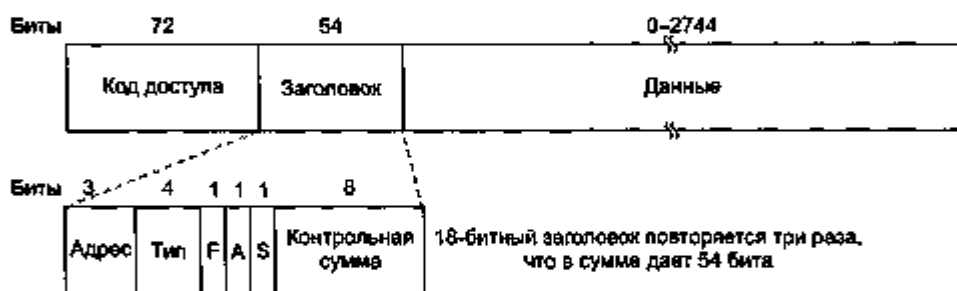
Рис. 4.34. Типичный информационный кадр Bluetooth
