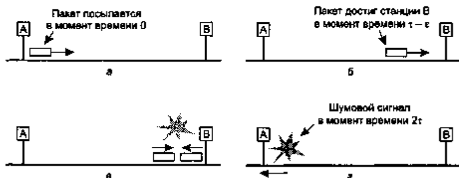
Рис. 4.17. Обнаружение столкновения может занять 2t
