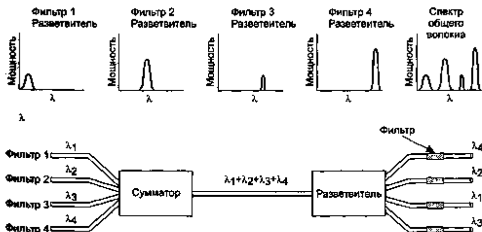
Рис. 2.28. Уплотнение с разделением длины волны
