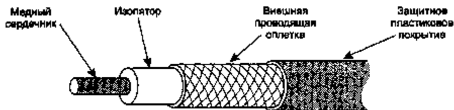
Рис. 2.3. Коаксиальный кабель
