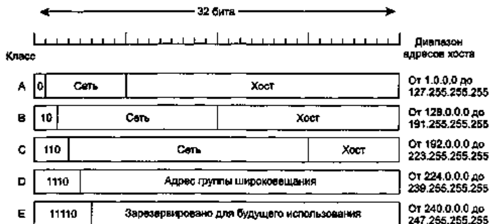
Рис. 5.48. Форматы IP-адреса
