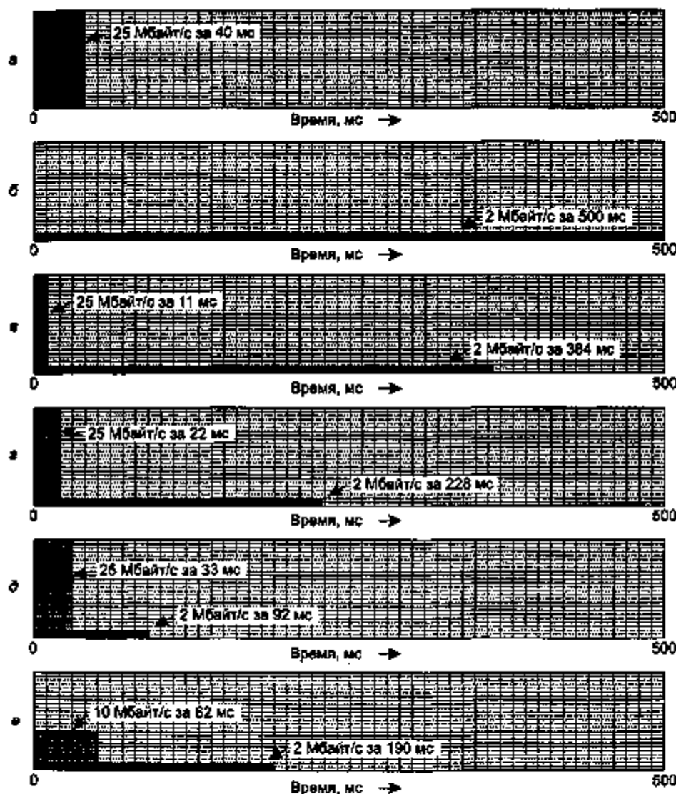
Рис. 5.20. Вход дырявого ведра (а); выход дырявого ведра (б); выход маркерного ведра емкостью 250 Кбайт (в), 500 Кбайт (г) и 750 Кбайт (д); выход маркерного ведра емкостью 500 Кбайт на входе дырявого ведра со скоростью протекания 10 Мбайт/с (е)
