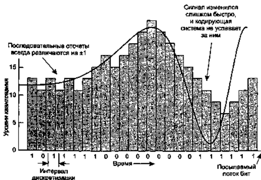
Рис. 2.30. Дельта-модуляция
