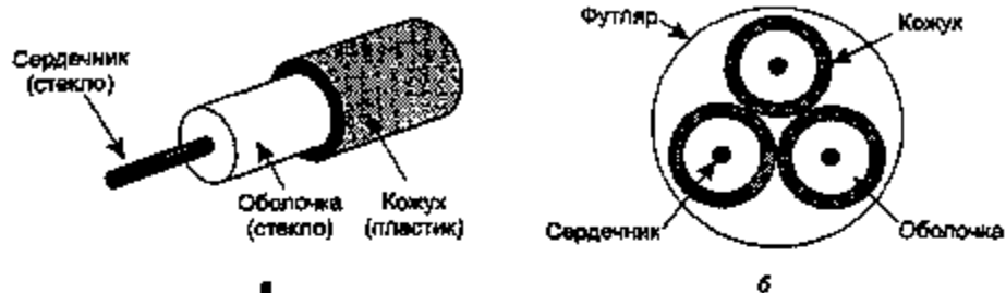
Рис. 2.6. Вид одиночного волокна сбоку (а); поперечное сечение трехжильного кабеля (б)
