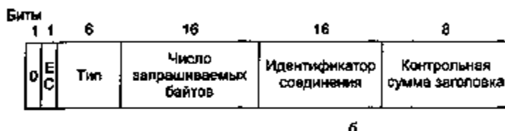
Рис. 4.31. Обычный кадр (а); кадр запроса канала (б)
