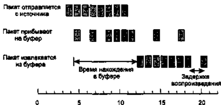
Рис. 5.27. Сглаживание выходного потока путем буферизации пакетов
