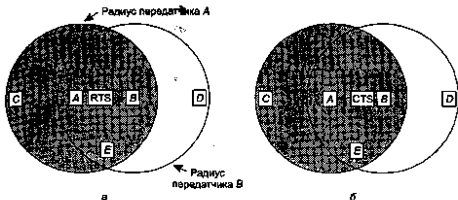
Рис. 4.12. Протокол MACA: станция A посылает кадр RTS станции B (а); станция B отвечает кадром CTS станции A (б)
