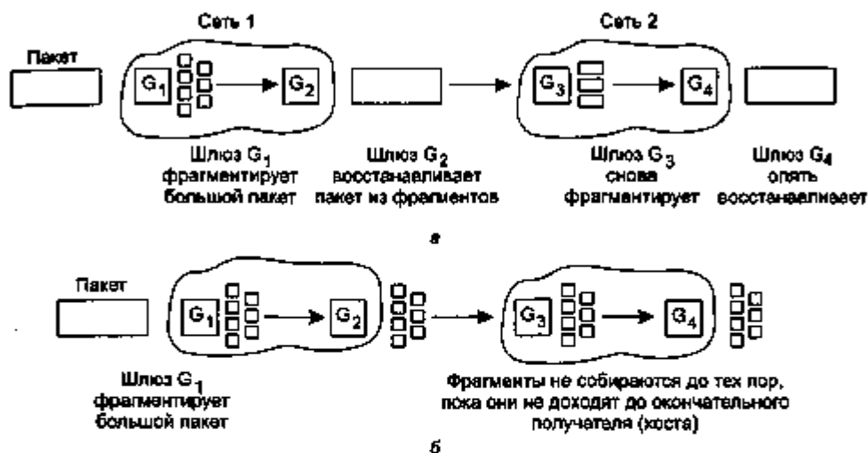
Рис. 5.44. Прозрачная фрагментация (а); непрозрачная фрагментация (б)
