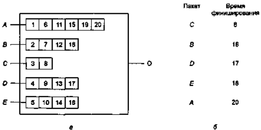
Рис. 5.31. Маршрутизатор с пятью очередями пакетов для линии O (а); время окончания сканирования для пяти пакетов (б)
