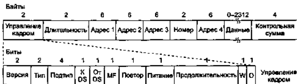
Рис. 4.27. Информационный кадр стандарта 802.11
