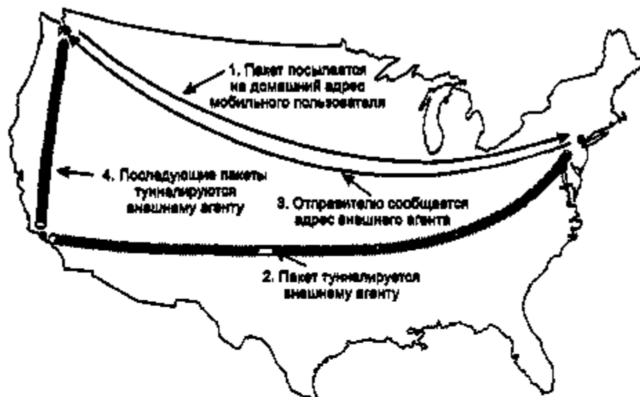
Рис. 6.17. Маршрутизация пакетов мобильным хостам
