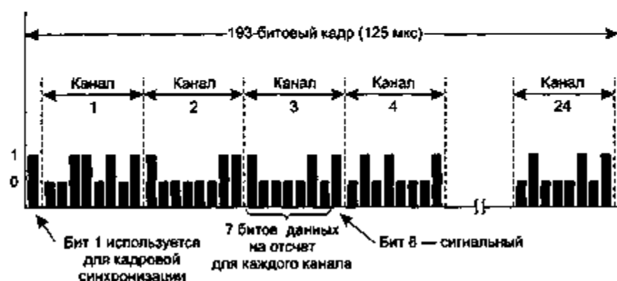
Рис. 2.29. Носитель T1 (1,544 Мбит/с)
