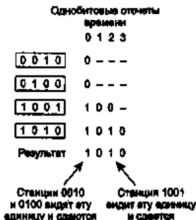
Рис. 4.7. Протокол с двойным обратным отсчетом. Прочерк означает молчание
