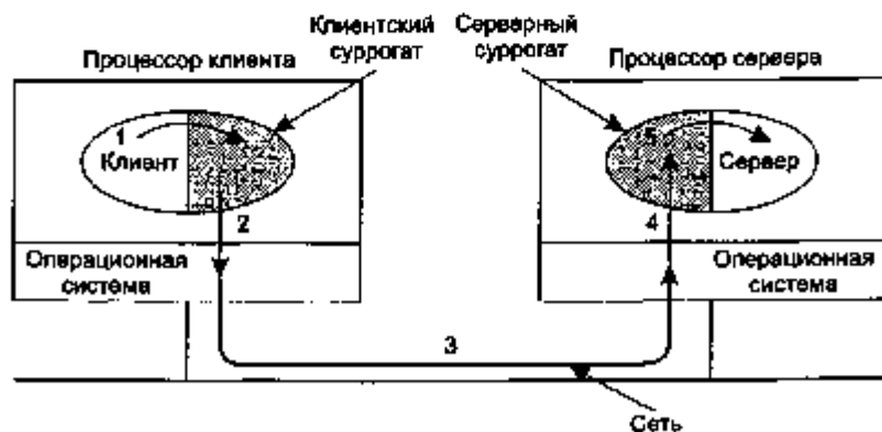
Рис. 6.16. Этапы выполнения удаленного вызова процедуры. Заглушки затенены
