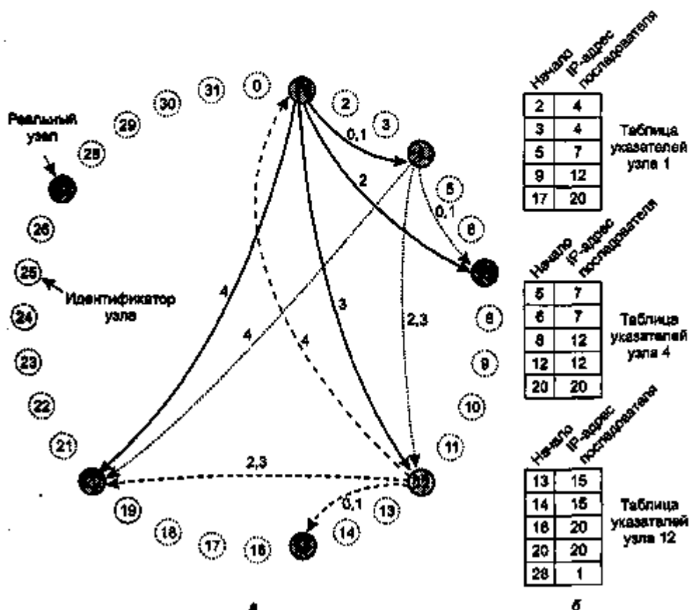
Рис. 5.22. Набор из 32 идентификаторов узлов, выстроенных по кругу (а). Закрашенные кружочки соответствуют реальным узлам. Дугами обозначены указатели с узлов 1, 4 и 12. Подписи на дугах соответствуют индексам таблицы. Примеры таблиц указателей (б)
