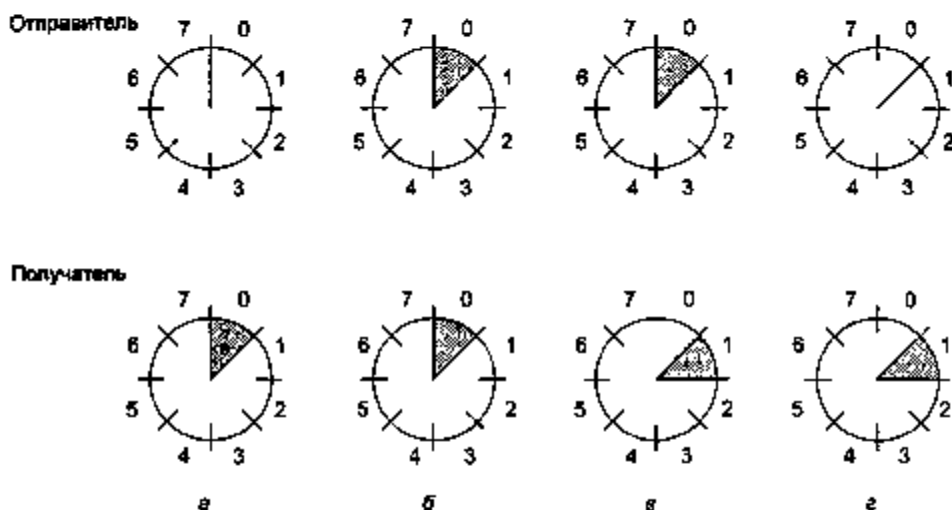
Рис. 3.9. Скользящее окно размера 1 с 3-битовым порядковым номером: начальная ситуация (а); после отправки первого кадра (б); после приема первого кадра (в); после приема первого подтверждения (г)
