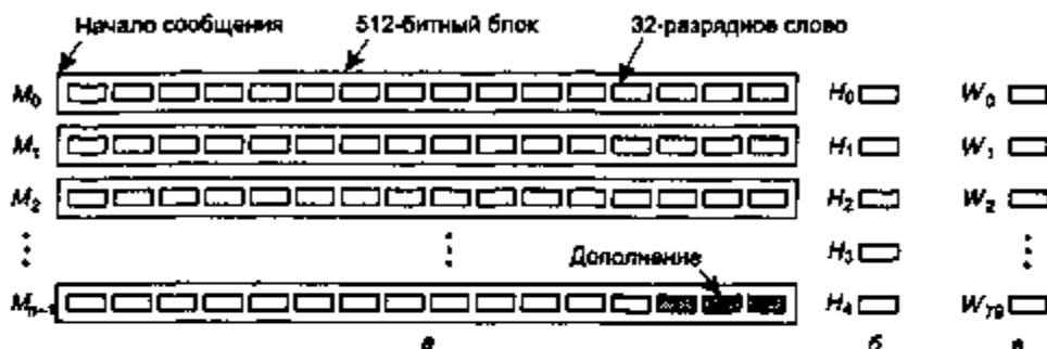
Рис. 8.19. Сообщения, дополненное до размера, кратного 512 битам (а); выходные переменные (б); массив слов (в)
