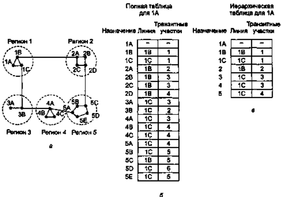
Рис. 5.13. Иерархическая маршрутизация
